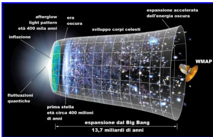
ESPANSIONE DEL BIG-BANG
